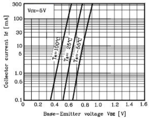
Fig. 2 I_C - V_{BE}
