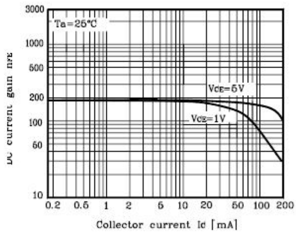
Fig. 4 h_{FE} - I_C
