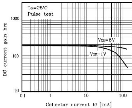
Fig. 4 h_{FE} - I_C
