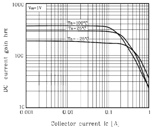
Fig. 6 h_{FE} - I_C
