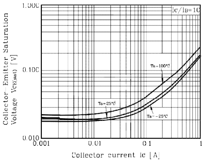
Fig. 5 I_C - V_{CE}
