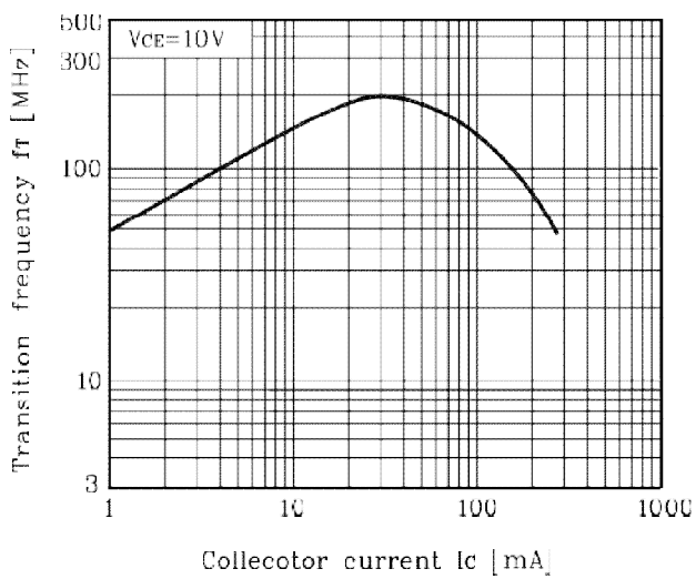
Fig. 5 f_T - I_C
