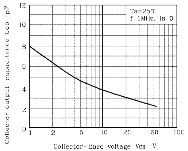
Fig. 6 C_{ob} - V_{CB}
