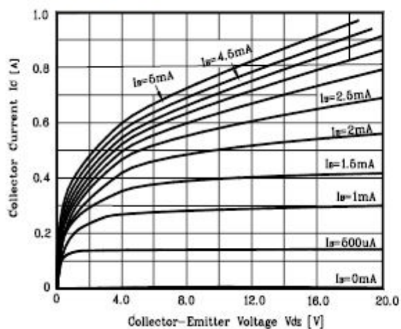
Fig. 5 I_C - V_{CE}
