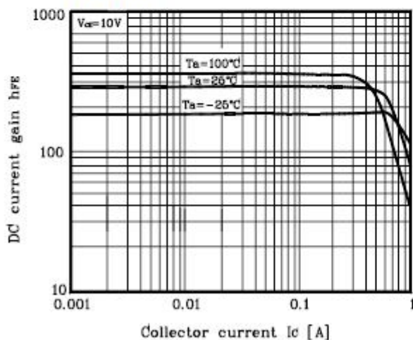
Fig. 9 h_{FE} I_C
