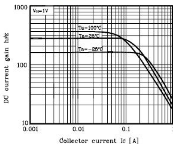
Fig. 6 h_{FE} - I_C
