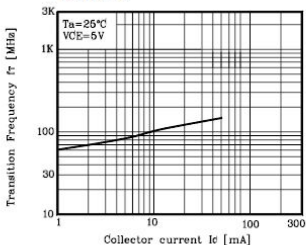
Fig. 11 f_T - I_C
