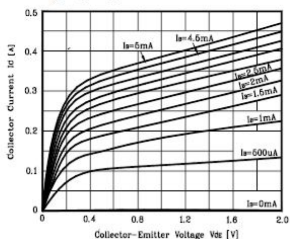
Fig. 4 I_C - V_{CE}
