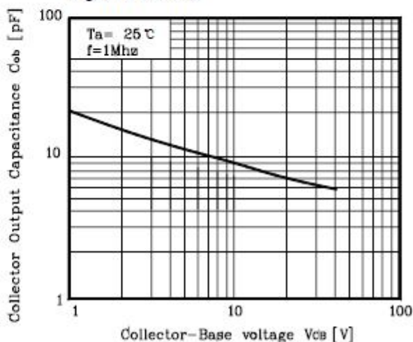
Fig. 10 C_{ob} - V_{CB}
