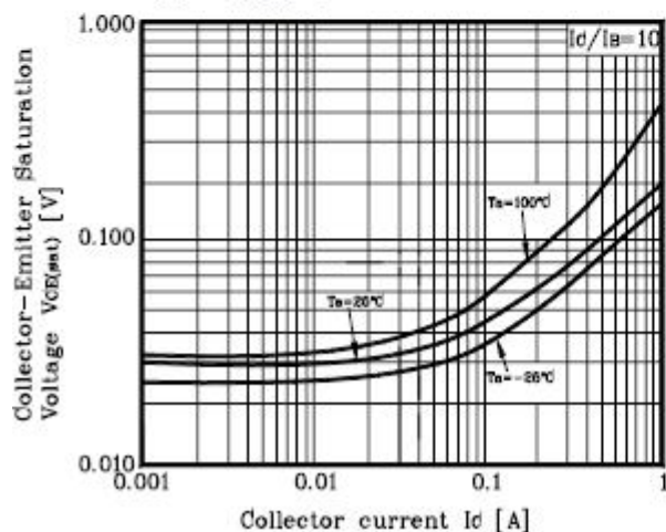
Fig. 3 V_{CE(sat)} - I_C
